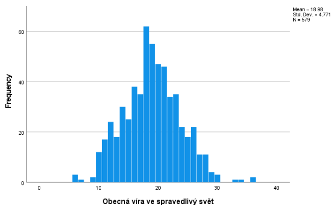
Graf 3 - Rozložení proměnné podpora trestu smrti
