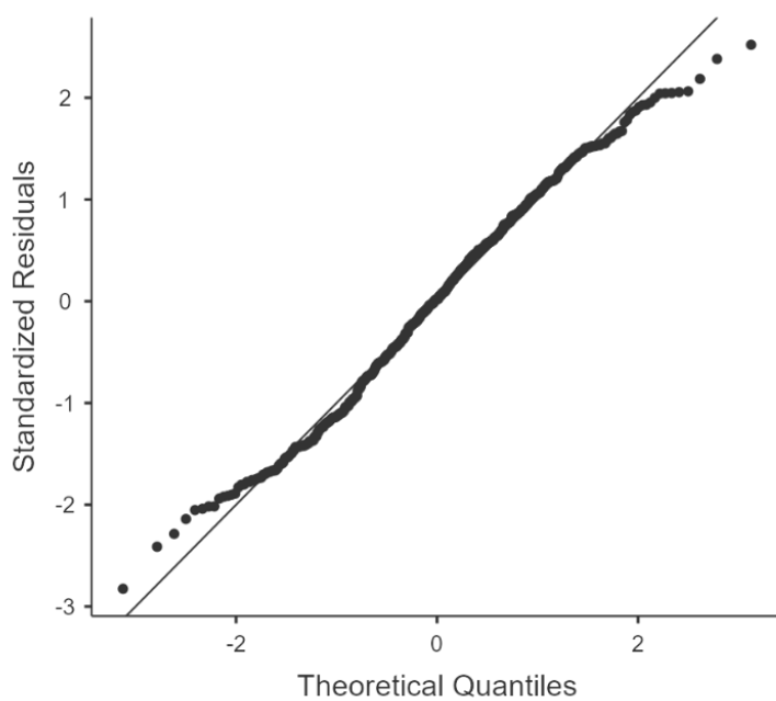
Graf 6 - Q-Q graf rozložení standardizovaných reziduí
