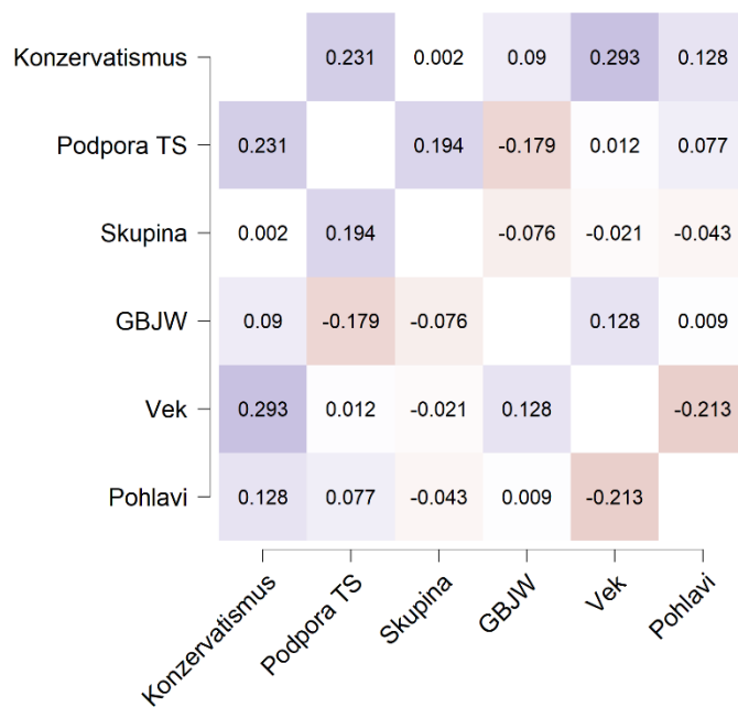
Graf 5 - Heat mapa korelací proměnných
