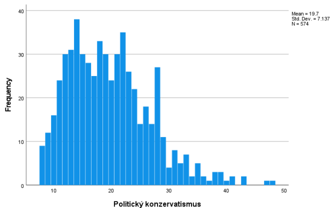
Graf 4 - Rozložení proměnné politický konzervatismus
