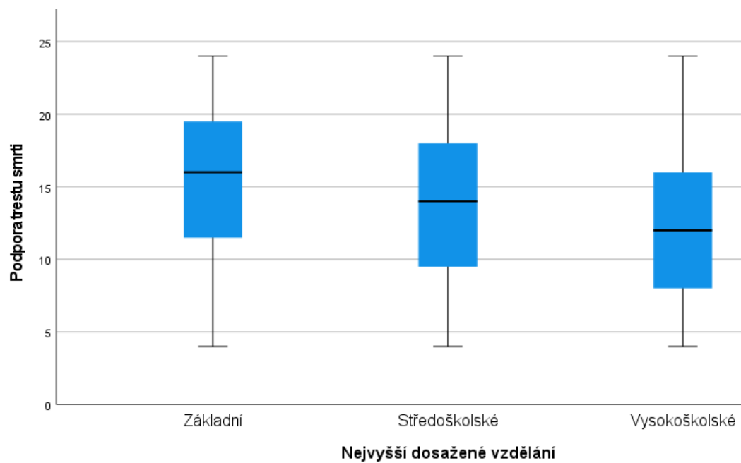
Graf 10 - Boxploty (s CI) míry podpory trestu smrti pro nejvyšší dosažené vzdělání
